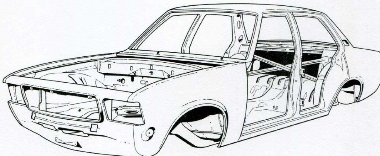
Rohkarosserie der 4 türigen Limousine
