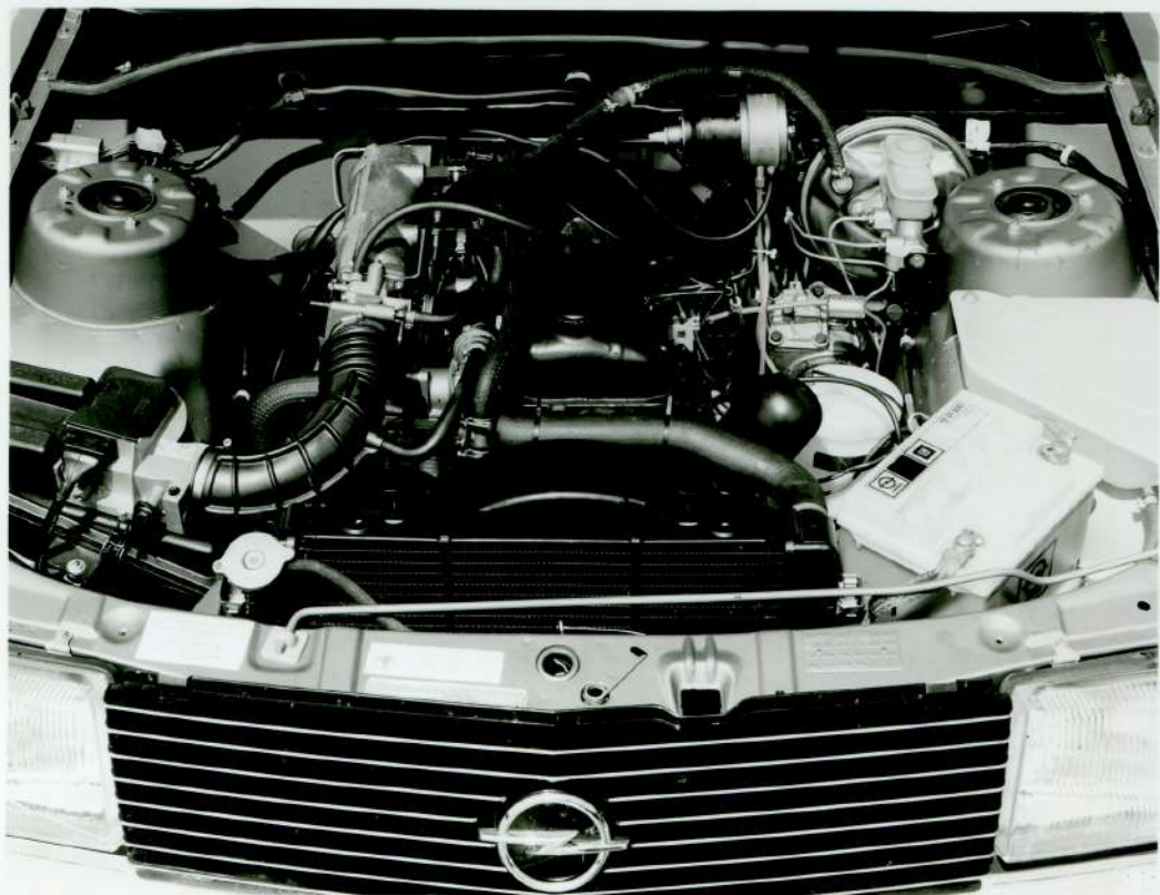
Opel Rekord 2,0 L-E Motor
