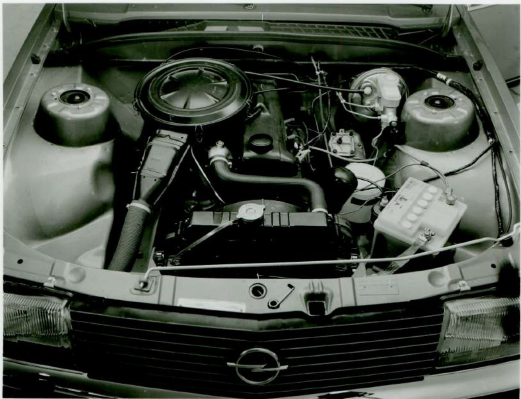
Opel Rekord, Vergasermotor
