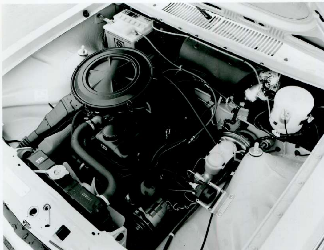
Opel Kadett Berlina, 1,6 L-S Motor
