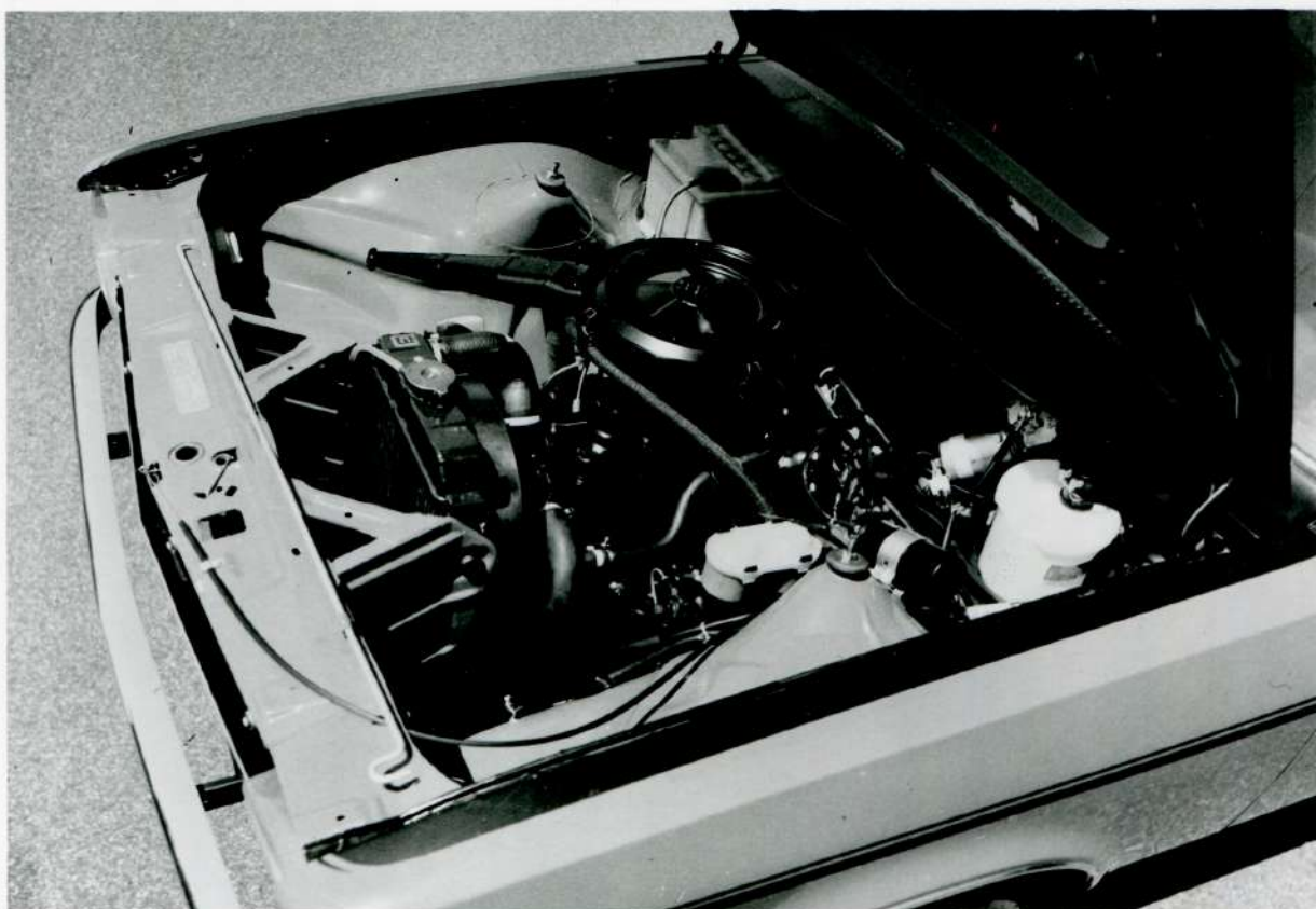
Opel Kadett SR, Motorraum
